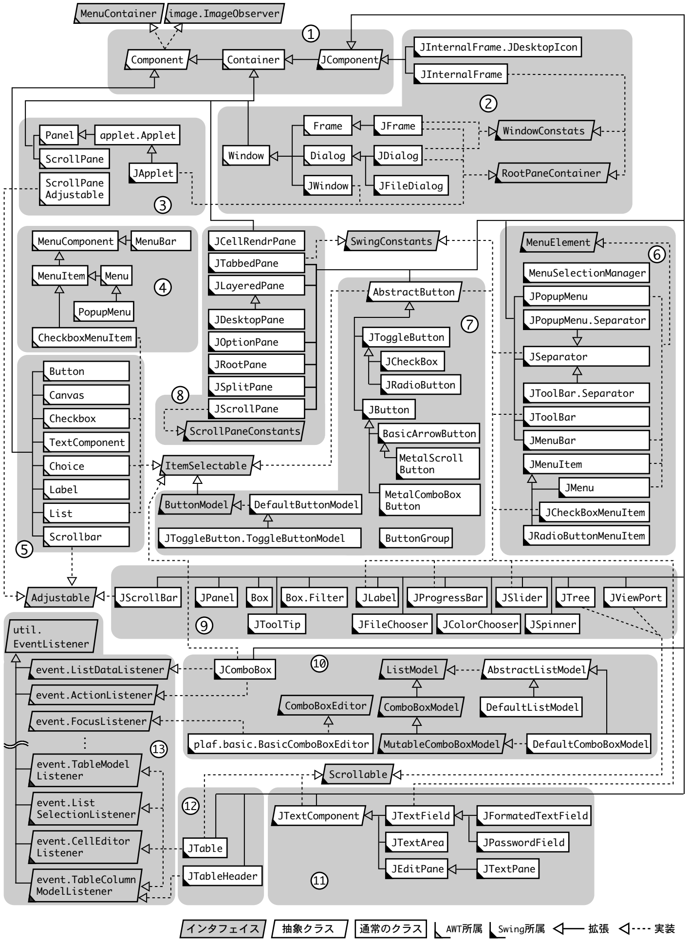
Fig. 5 [GUIコンポーネントの主な実装・継承関係]
